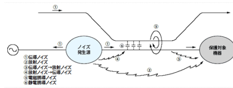
図1 ノイズ発生と進入経路（出典：富士電機 HP）
