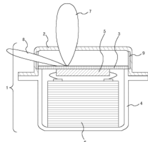
図3 ミリ波レーダー(断面図)から送信されるサイドロブの影響 (出典：特開 2004-77399)
